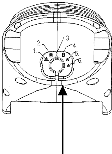
Vridströmställare
