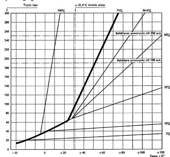
Tryck-temperaturdiagram för kolsyrebehållare vid olika fyllningsgrader
